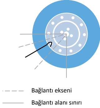
ÇELİK TEKERLEKLERİN SABİTLENMESİ Her tekerleğe bir düz kanca ile kemer bağlanır
