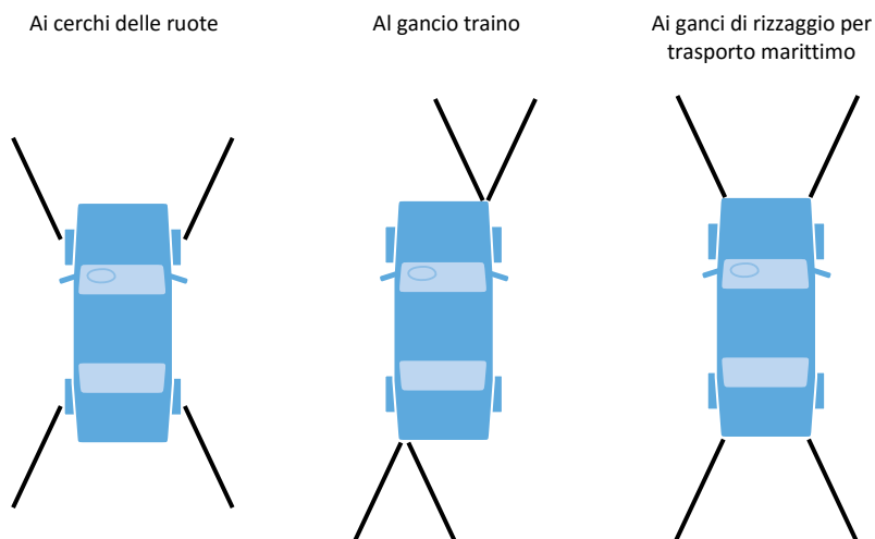
Stivaggio longitudinale
